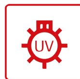
Polymérisation Polymerization
